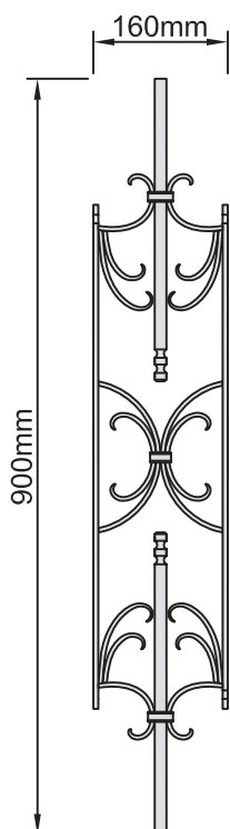
Geländerstab Nr. 1716-GD
