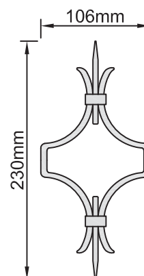
Distanzelement Nr. 1727-GD
