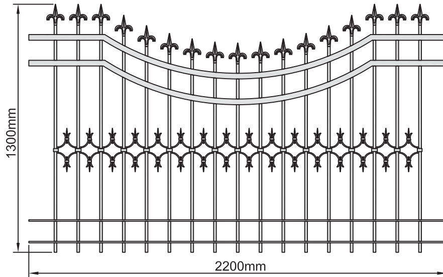
Zaunfeld Nr. 1774-GD
