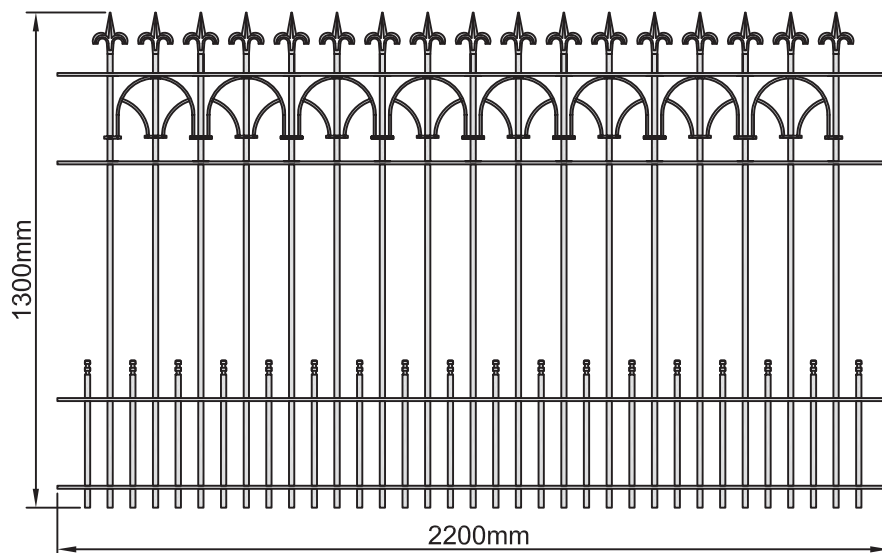
Zaunfeld Nr. 1775-GD
