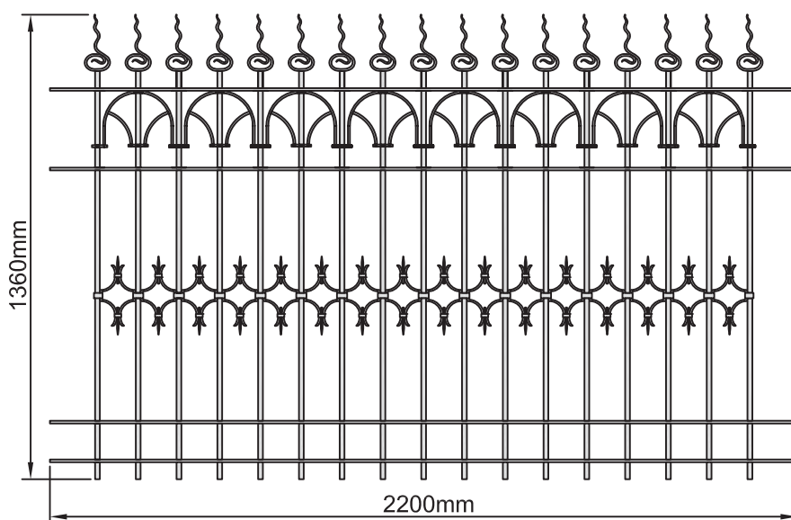
Zaunfeld Nr. 1771-GD
