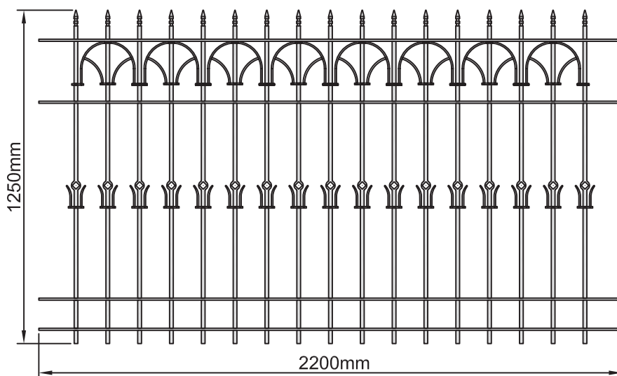
Zaunfeld Nr. 1770-GD
