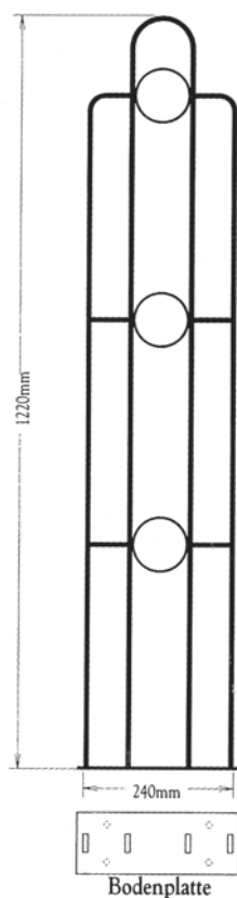
Art.-Nr. 1690 Gewicht: 12,0 kg Material: 30/8 mm Maßstab 1:10 inkl. Bodenplatte
