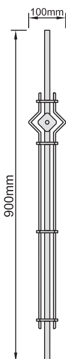
Geländerstab Nr. 1719-GD
