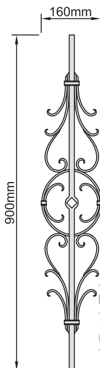
Geländerstab Nr. 1717-GD
