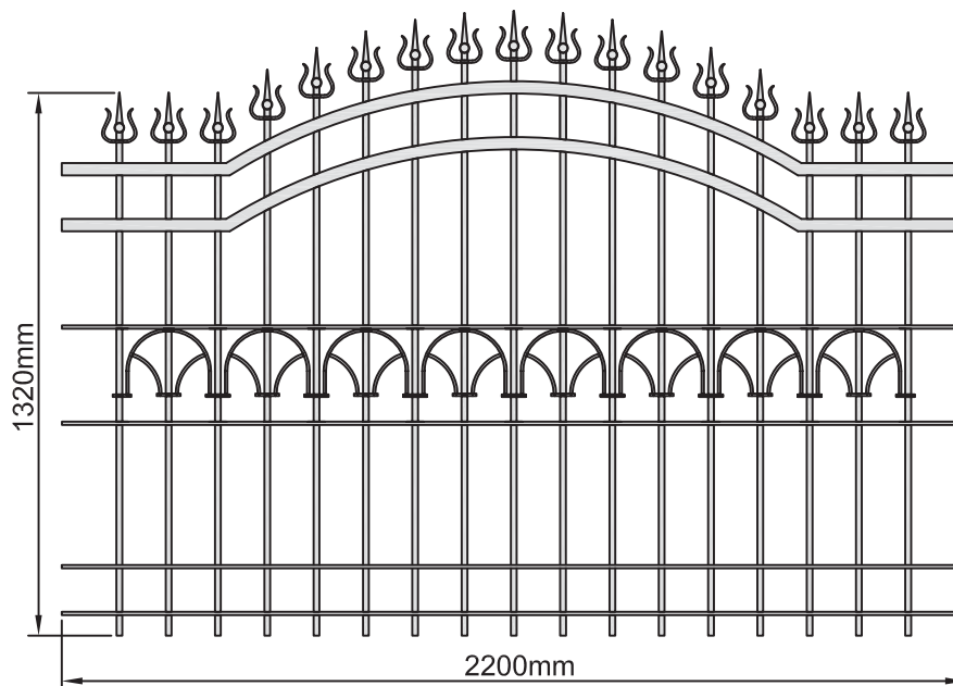
Zaunfeld Nr. 1776-GD
